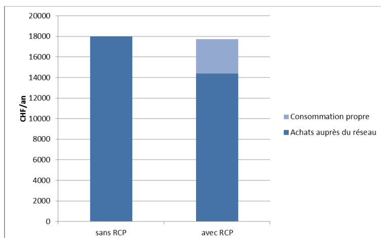
Illustration 8 : Grand immeuble d'habitation avec une faible consommation électrique – coûts annuels d'achat d'énergie sans et avec RCP
