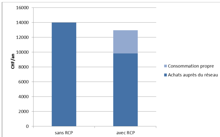
Illustration 7 : Petit immeuble d'habitation – coûts annuels d'achat d'énergie sans et avec RCP
