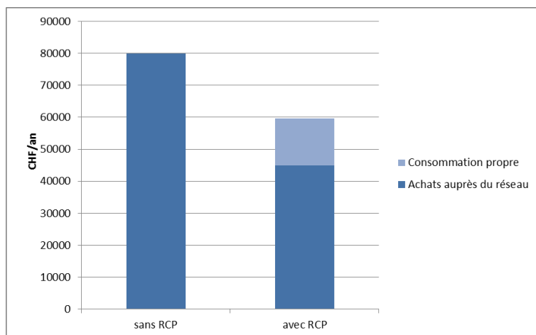
Illustration 9 : Grand immeuble d'habitation avec une consommation électrique moyenne – coûts annuels d'achat d'énergie sans et avec RCP
