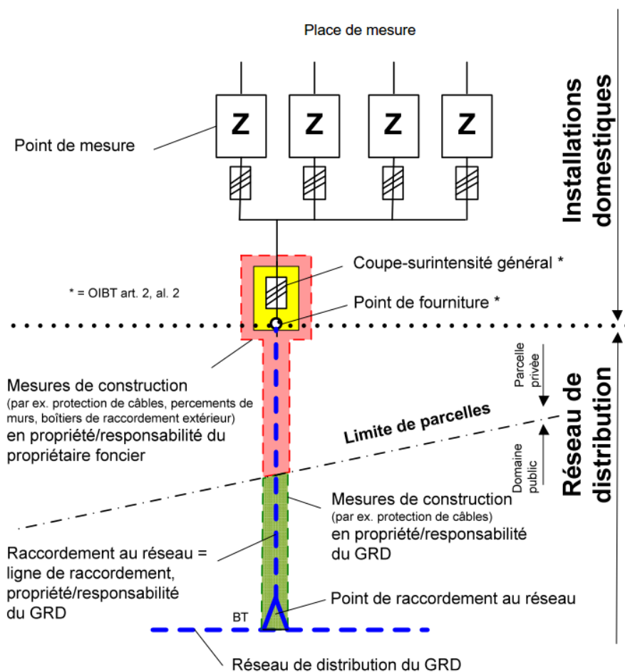
Illustration 3 : Représentation du raccordement au réseau, source : bulletin.ch 10 / 2017, article d'Olivier Stössel
